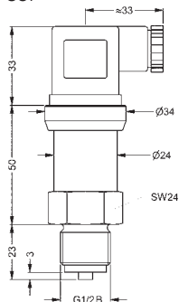
Connection G \frac{1}{2} B EN 837
