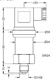
Connection G \frac{1}{4} B EN 837
